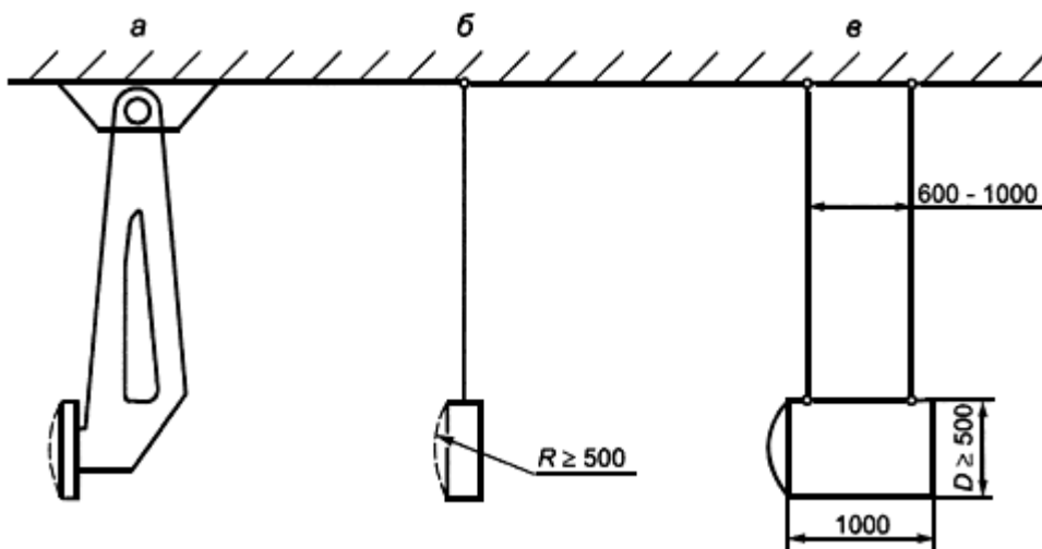
а - жесткая подвеска; б - гибкая одиночная подвеска; в - гибкая двоянная подвеска
